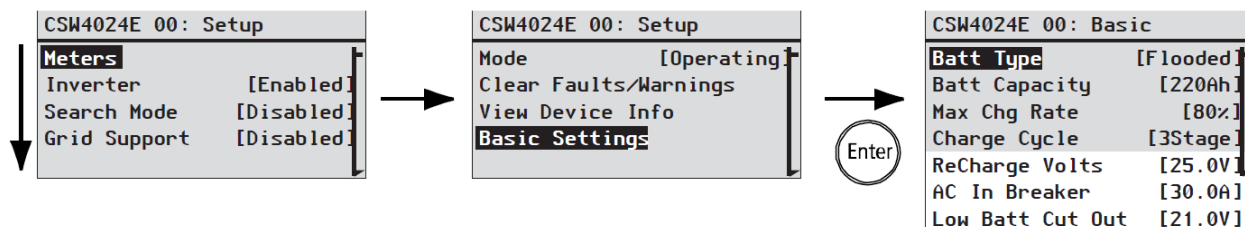
Рисунок 4-1 Выбор основных настроек
