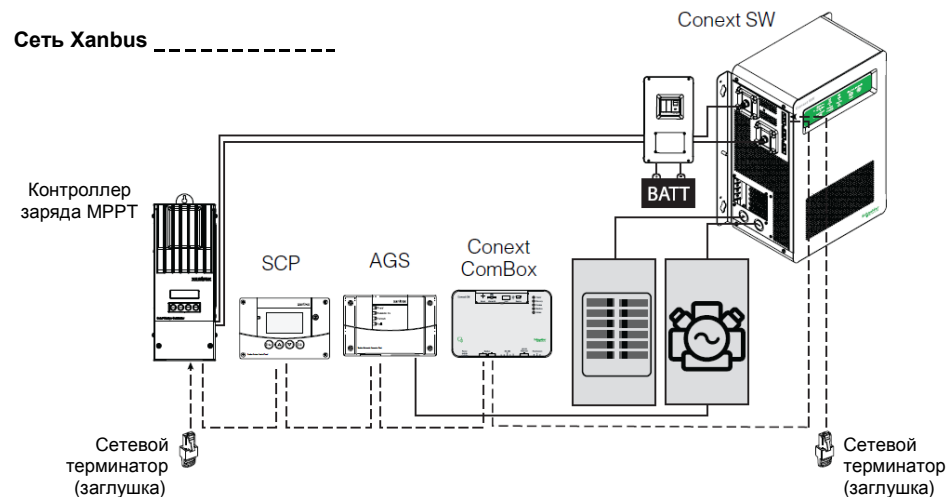
Рисунок 2-1 Компоненты системы Ханбус
